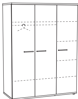
K3 150 x 200 x 64 cm
