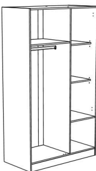
AR2P : L101 x H182 x P51 cm
